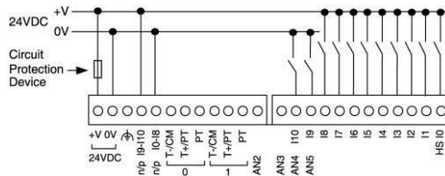
Câblage d'entrée (I0-I8), pnp, (I9-I10), npn
