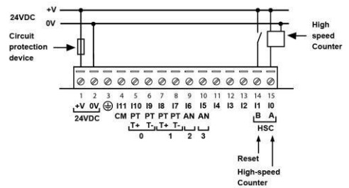
Câblage d'entrée HSC
