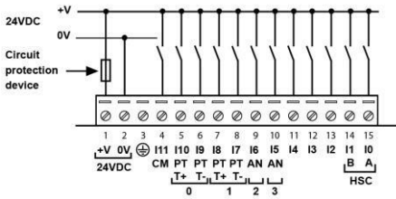
Câblage d'entrée
